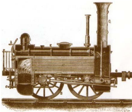
Locomotive Stephenson vue en coupe
